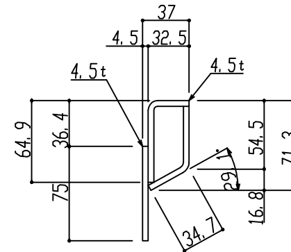
端上げ材詳細図
